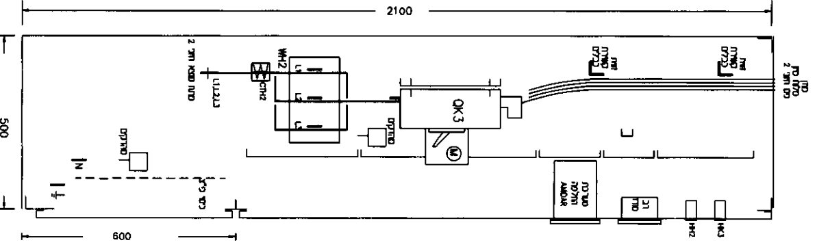
חוקן צד A-A
