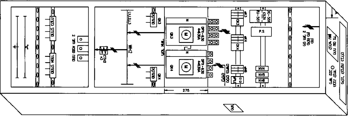
סכנה הלוח - חזית פנימית
